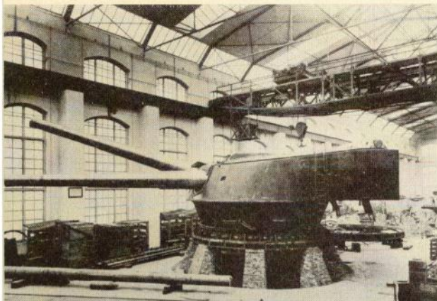
Ett av "Sverige-tornen" under montage i Kanonverkstaden. Foto Pontus Andersson.
