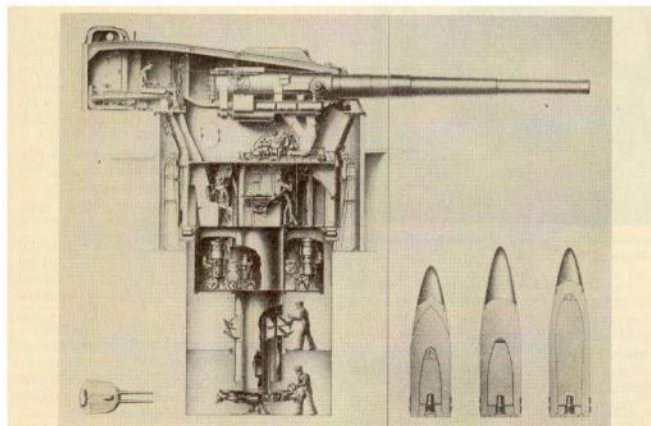
Sektion av ett 28 cm dubbeltorn, stående ammunitionslösar m. m. Längst ned t. h. tre olika granater. Originalteckningen är utsålld i Statens Sjökrigshistoriska Múzeum.
